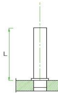
COLONNA TIPO ESTRAIBILE CE REMOVABLE PIN CE
